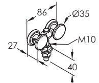
No. 56KN or No. 56KS HANGER
